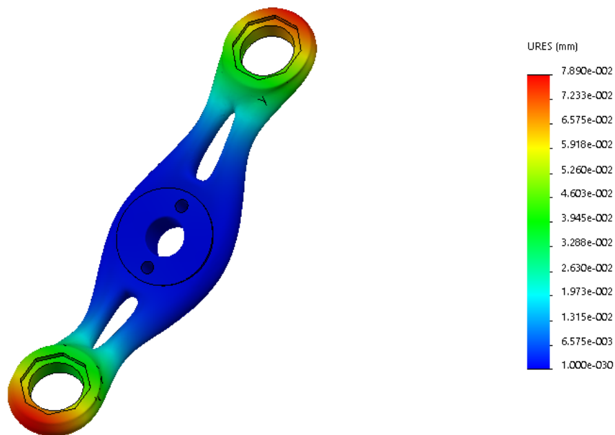
Figura 9 - schema di carico 2, vista tergale, deformata amplificata
