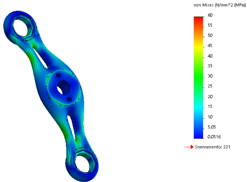
Figura 10 - schema di carico 3, vista frontale, distribuzione delle tensioni superficiali secondo Von-Mises
