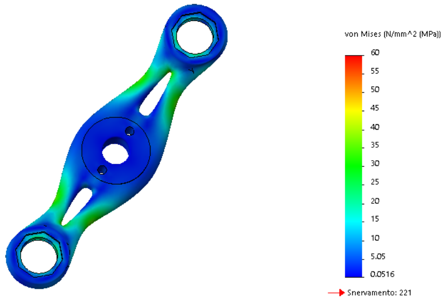
Figura 12 - schema di carico 3, vista tergale, distribuzione delle tensioni superficiali secondo Von-Mises
