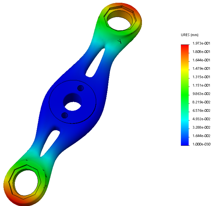
Figura 5 - schema di carico 1, vista tergale, deformata amplificata
