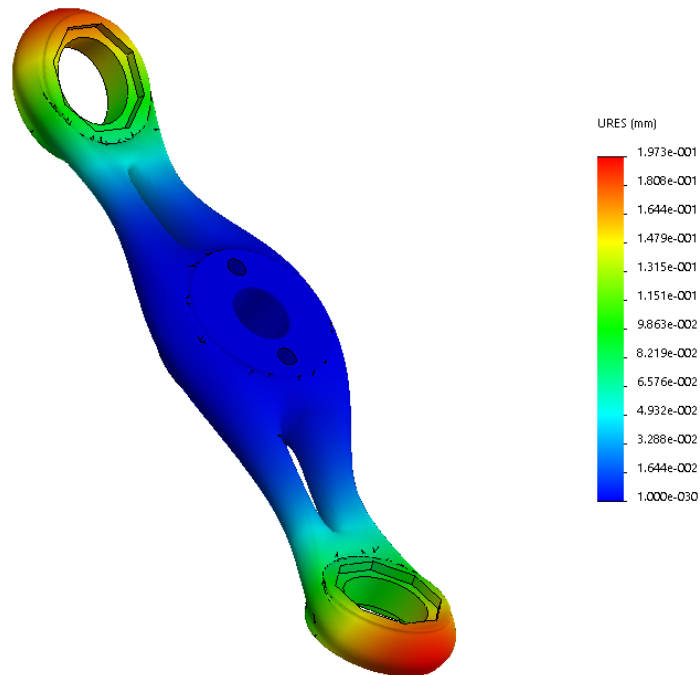
Figura 3 - schema di carico 1, vista frontale, deformata amplificata
