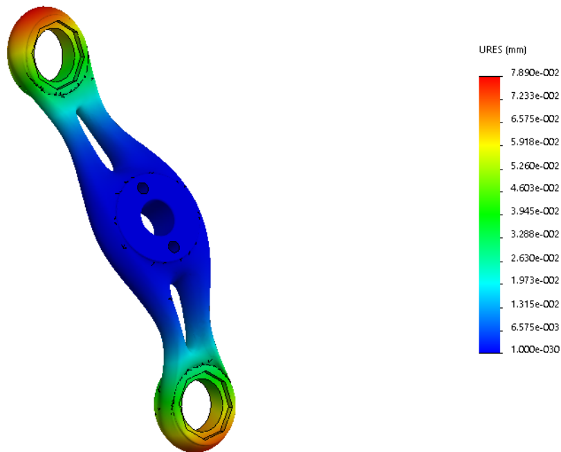
Figura 7 - schema di carico 2, vista frontale, deformata amplificata
