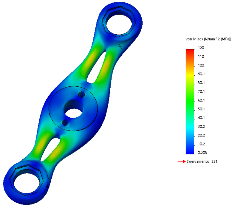
Figura 4 - schema di carico 1, vista tergale, distribuzione delle tensioni superficiali secondo Von-Mises
