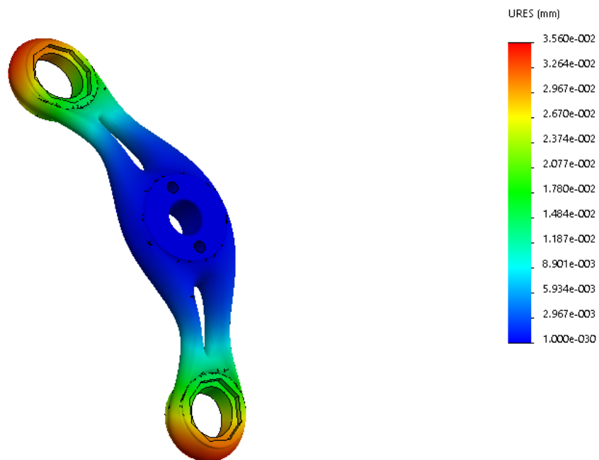
Figura 11 - schema di carico 3, vista frontale, deformata amplificata
