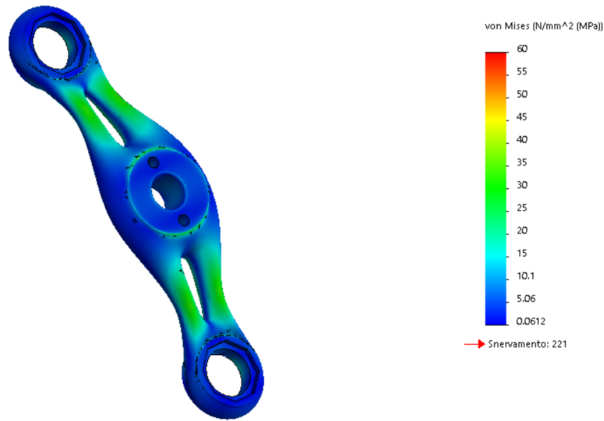
Figura 6 - schema di carico 2, vista frontale, distribuzione delle tensioni superficiali secondo Von-Mises
