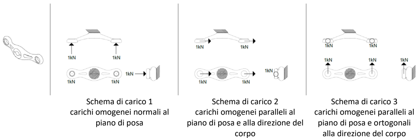
Figura 1 – schemi di carico
