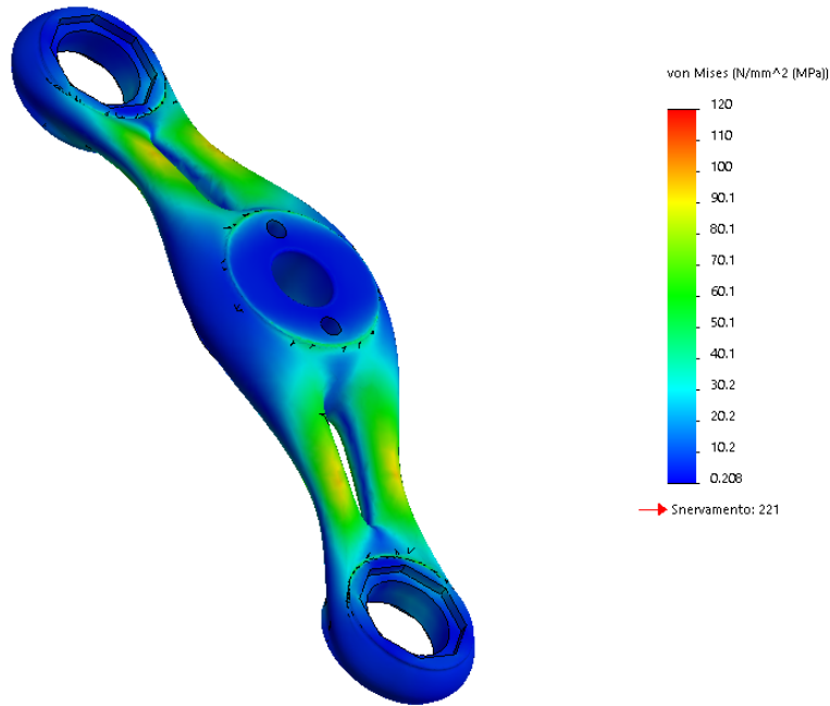
Figura 2 - schema di carico 1, vista frontale, distribuzione delle tensioni superficiali secondo Von-Mises
