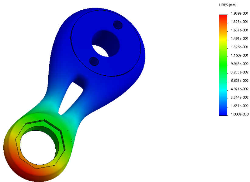
Figura 3 - schema di carico 1, vista frontale, deformata amplificata
