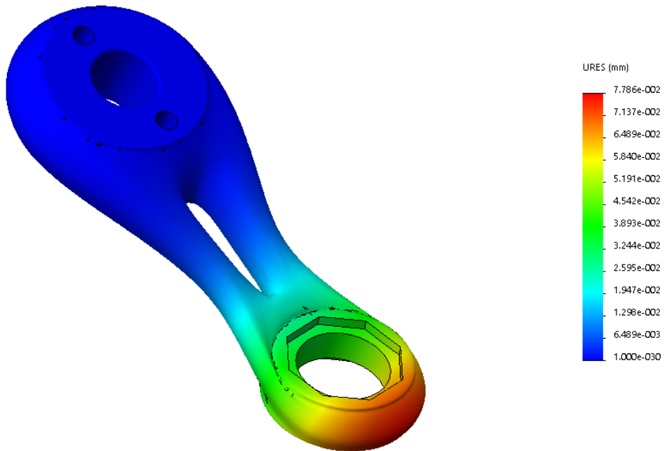
Figura 9 - schema di carico 2, vista tergale, deformata amplificata
