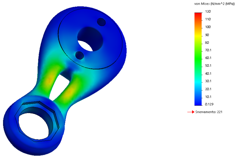
Figura 2 - schema di carico 1, vista frontale, distribuzione delle tensioni superficiali secondo Von-Mises
