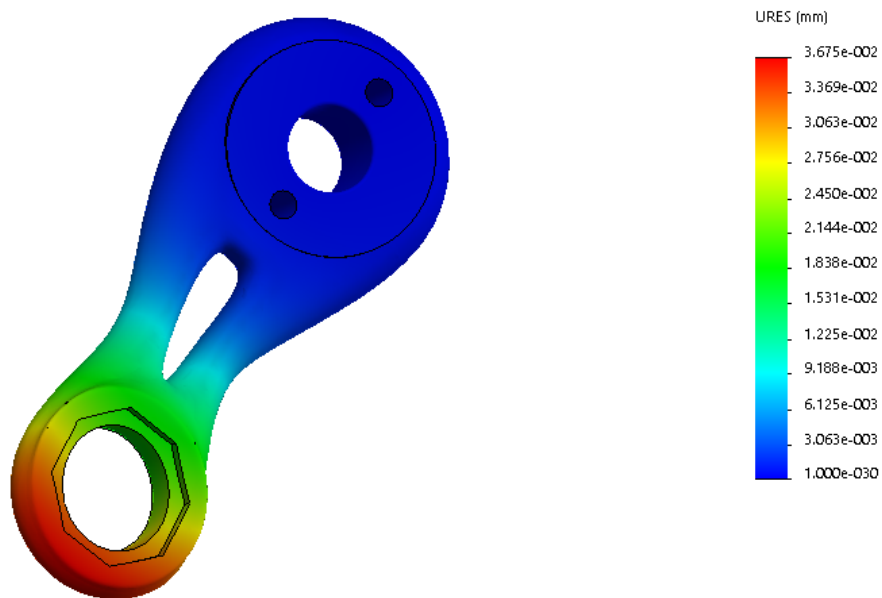
Figura 11 - schema di carico 3, vista frontale, deformata amplificata
