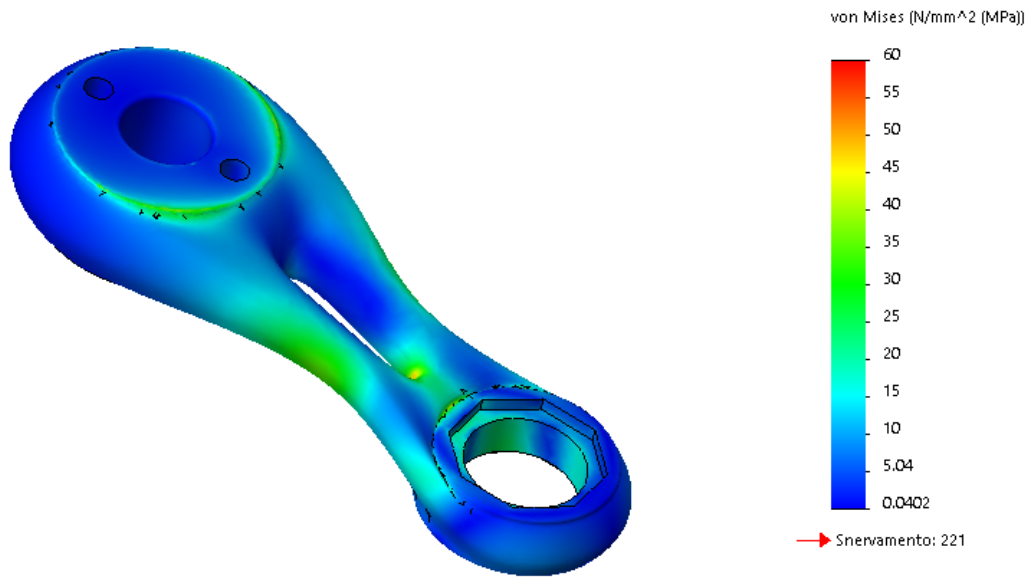
Figura 12 - schema di carico 3, vista tergale, distribuzione delle tensioni superficiali secondo Von-Mises
