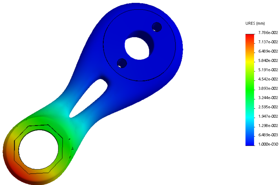
Figura 7 - schema di carico 2, vista frontale, deformata amplificata
