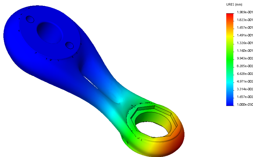
Figura 5 - schema di carico 1, vista tergale, deformata amplificata
