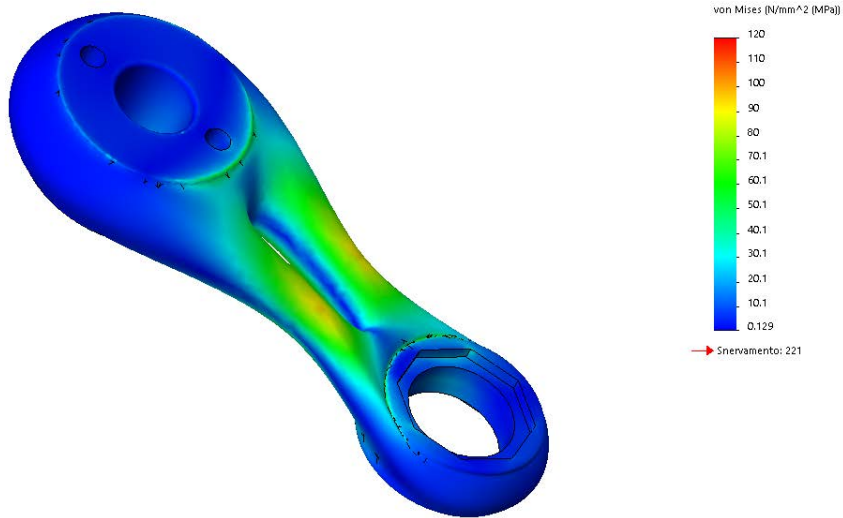
Figura 4 - schema di carico 1, vista tergale, distribuzione delle tensioni superficiali secondo Von-Mises
