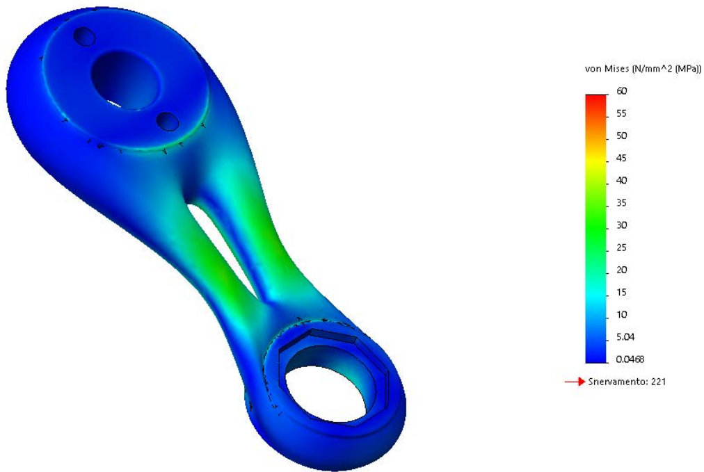
Figura 8 - schema di carico 2, vista tergale, distribuzione delle tensioni superficiali secondo Von-Mises
