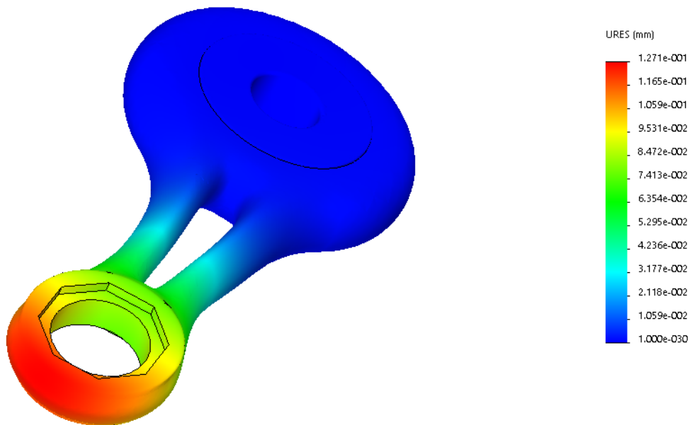
Figura 7 - schema di carico 2, vista frontale, deformata amplificata
