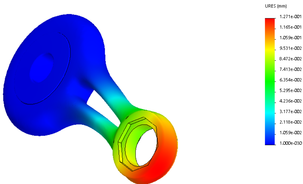
Figura 9 - schema di carico 2, vista tergale, deformata amplificata
