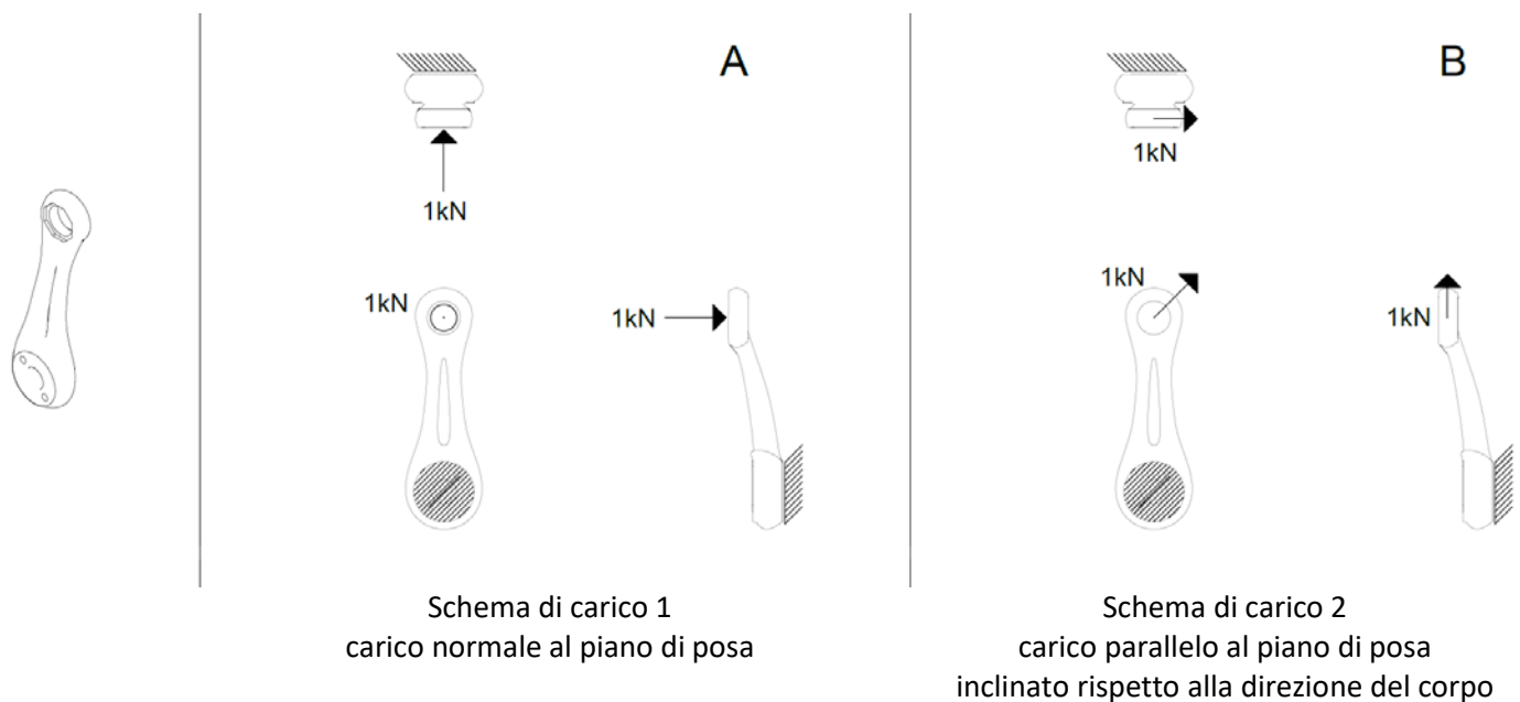
Figura 1 – schemi di carico
