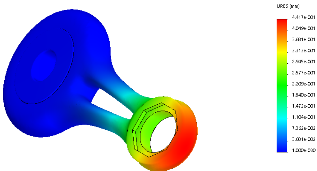
Figura 5 - schema di carico 1, vista tergale, deformata amplificata
