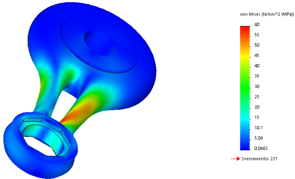
Figura 6 - schema di carico 2, vista frontale, distribuzione delle tensioni superficiali secondo Von-Mises
