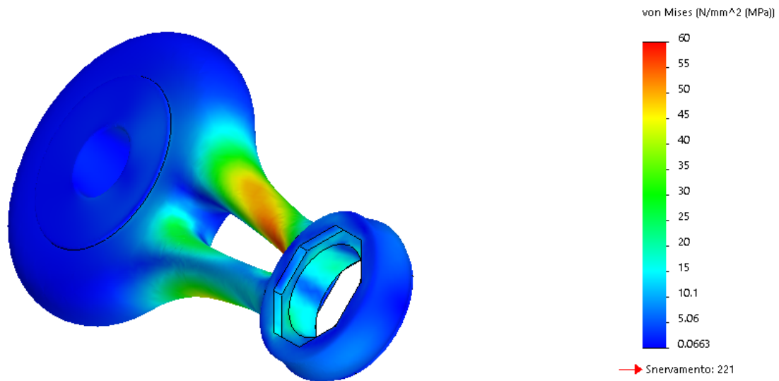
Figura 8 - schema di carico 2, vista tergale, distribuzione delle tensioni superficiali secondo Von-Mises
