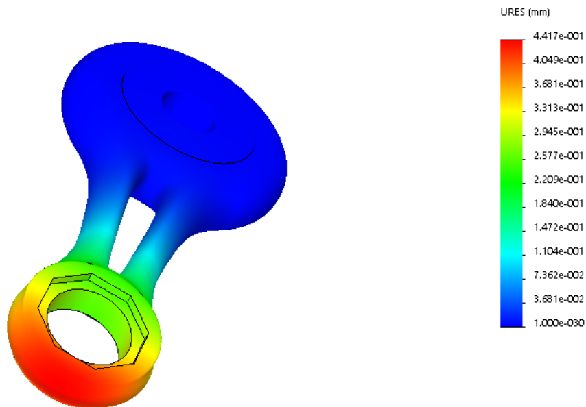
Figura 3 - schema di carico 1, vista frontale, deformata amplificata
