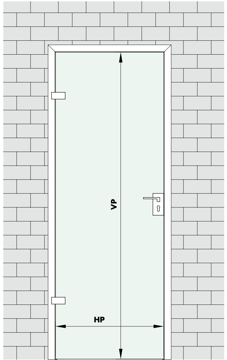
Dimensions du vantail en verre
