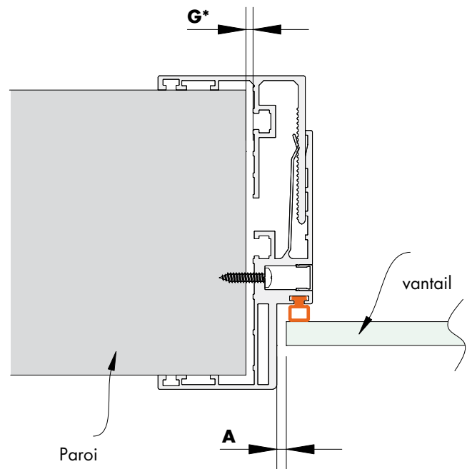
Dimensions du vantail en verre
