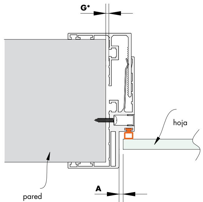
Dimensiones de la hoja de vidrio
