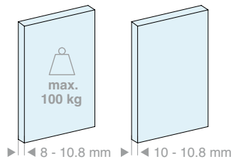
VERRE VANTAIL
