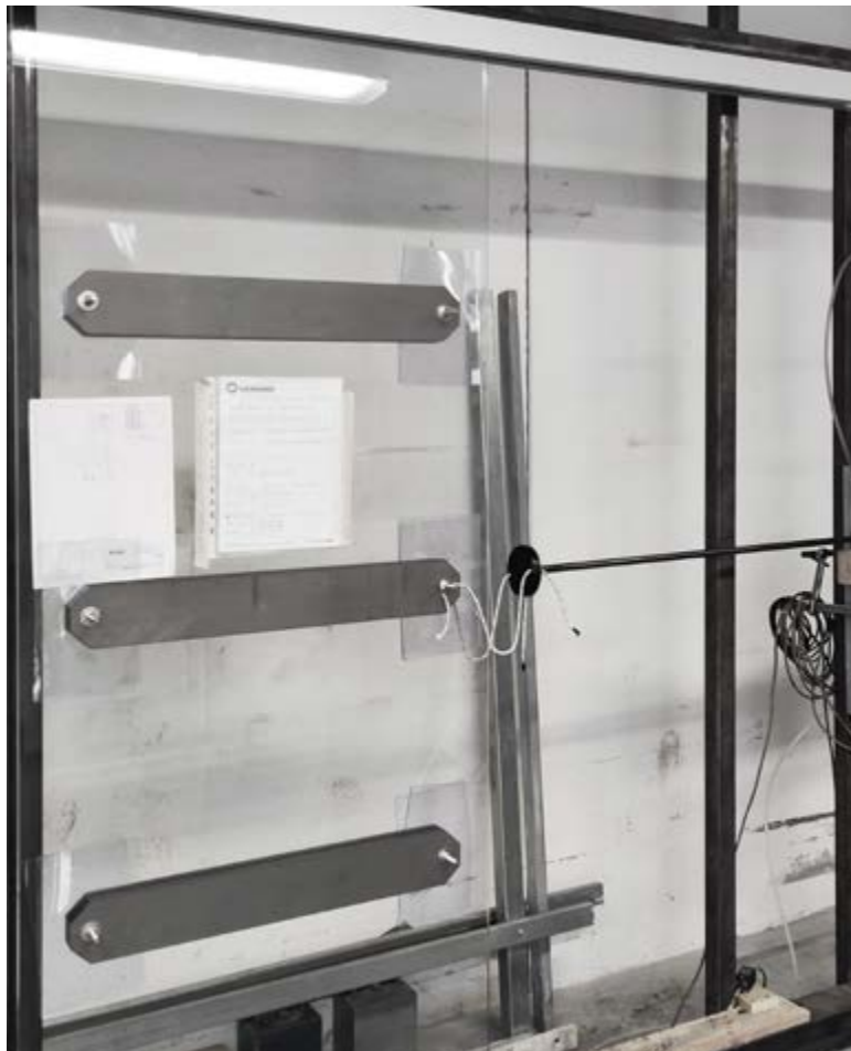
Performances testées jusqu'à 45 000 cycles d'ouverture et de fermeture
