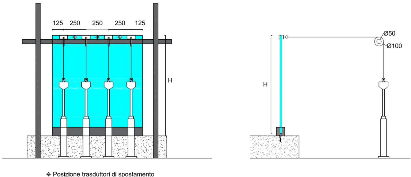
Figura 4.2 – Prova statica -schema sistema di prova – Vista frontale e laterale (misure in mm)
