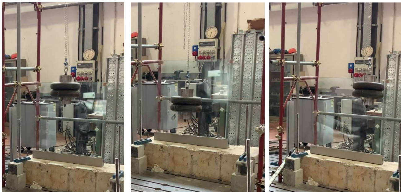
Figura 5.4 – SH- DF810ML-8T8I-2PVB– Impatto punti 1-2-3
