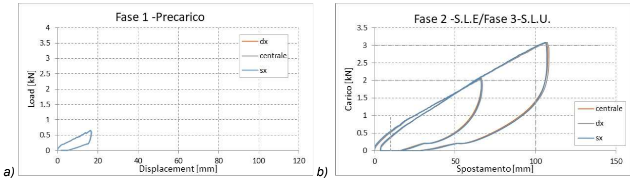
Figura 5.1 – Campione DF810ML-8T8I-2PVB -Curve carico-spostamento: Precarico e S.L.E ed S.L.U.
