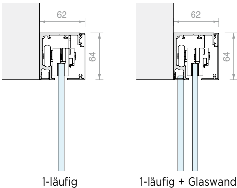
1-läufig
